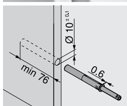
Усиленный TIP-ON, врезной
