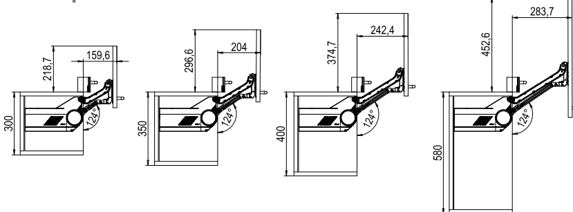
Рычаг 21L3200
