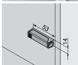
Стандартный TIP-ON в прямоугольном держателе
