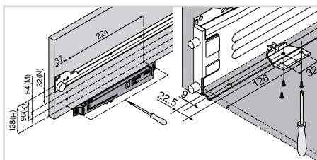
Установочные размеры для BLUMOTION
