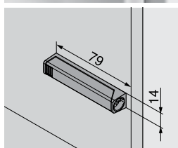
Усиленный TIP-ON в прямоугольном держателе
