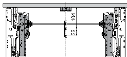
Механизм TIP-ON BLUMOTION, тип L1, L3, L5 (NL ≥ 350–650 мм)
