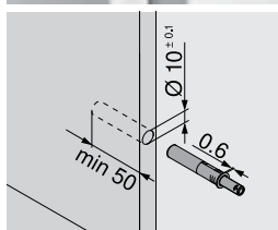
Стандартный TIP-ON, врезной
