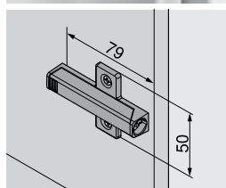
Усиленный TIP-ON в крестообразном держателе
