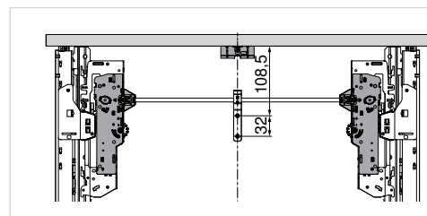
Механизм TIP-ON BLUMOTION, тип S0, S1 (NL < 350 мм)
